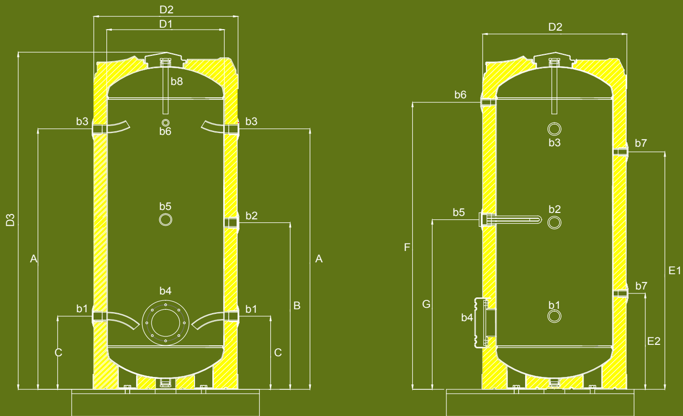
Skylight Akümülayon Tankı Boyut Tablosu Skylight Accumulation Size Spesification Table
