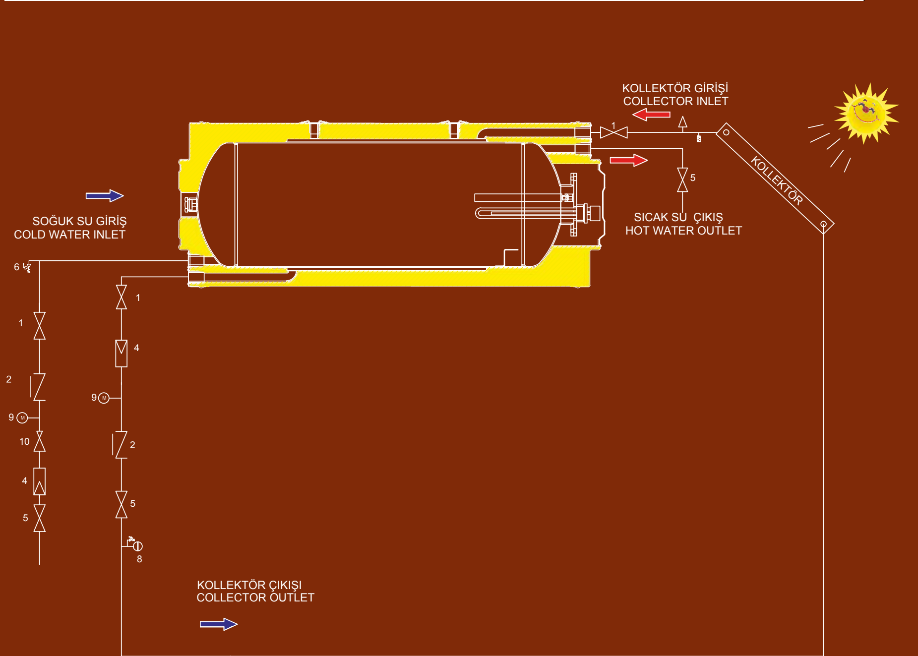
Daylight Yatık Basıncılı Boyler Bağlantı Şeması Daylight Horizontal Boiler Connection Scheme
